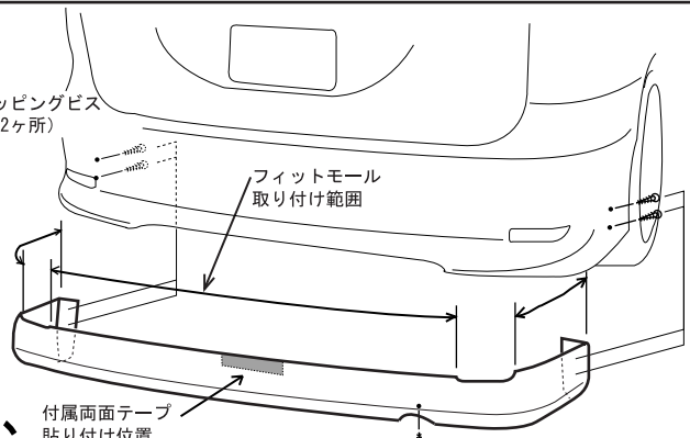
付属タッピングビス (左右各2ヶ所)
