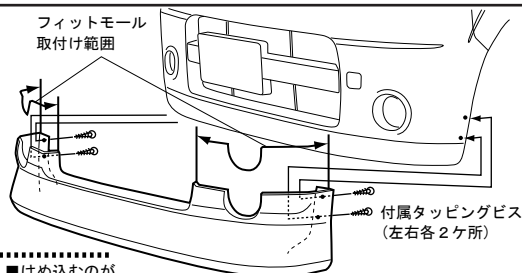
モール取付け図
