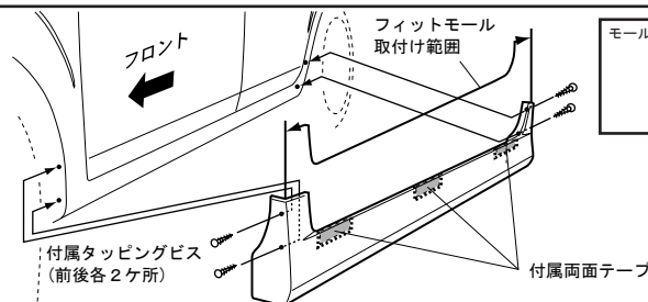
モール取付け図
