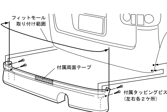
モール取付け図
