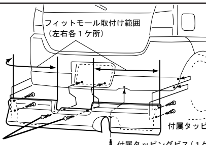
モール取付け図
