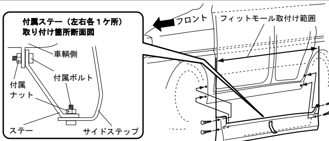
モール取付け図
